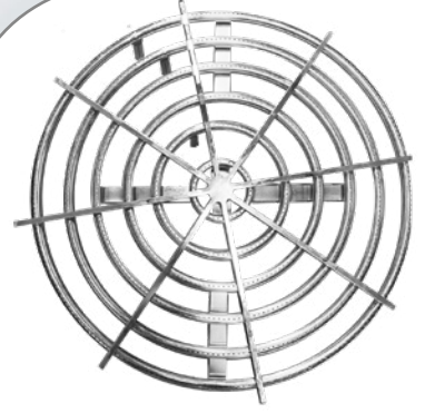
KUNAFE BRÜLÖR 6 RULMANLI
